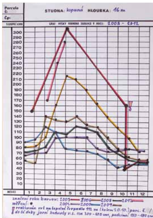
Měření hladiny vody v jedné studni ve Stříbrné Lhotě
