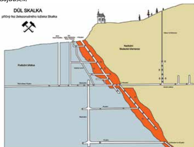
Ilustrační řez dolem, zdroj: Montánní společnost
