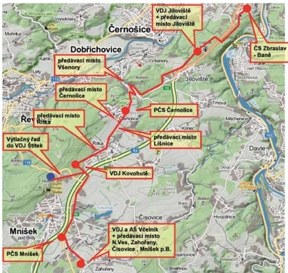
Trasa Regionálního vodovodního přivaděče pitné vody ze zbraslavských Baní do Mníšku pod Brdy i s důležitými technickými body
