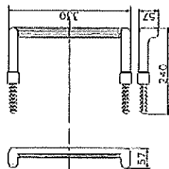
DETAILNÍ POHLED NA STUPAČLO "KASI"
