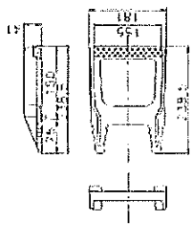
DETAILNÍ POHLED NA STUPAČLO DIN 1212 E
